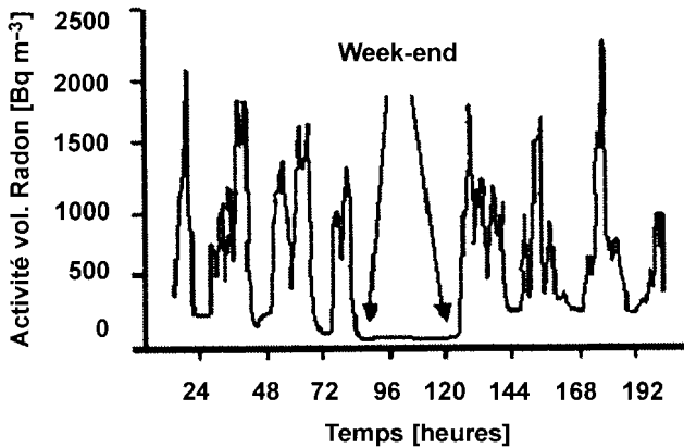
Figure 1 – Variation temporelle de l'activité volumique du radon dans une salle de soins d'une station thermale sur une période d'une semaine (d'après Lettner et al. , 1996).
