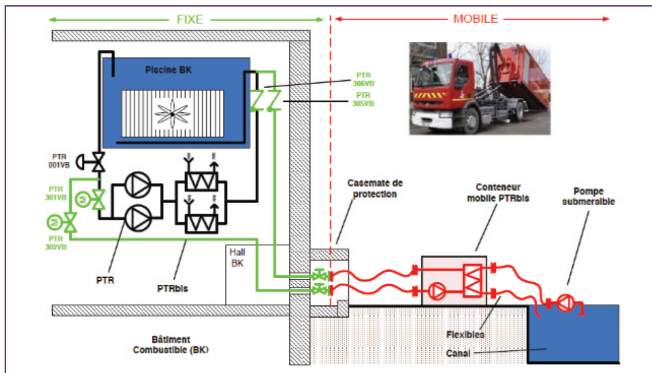
Figure 8. Schéma de principe du circuit de refroidissement mobile de la piscine combustible (PTR bis) (source : EDF SA - 2018 - Note de réponse aux objectifs du 4 e réexamen périodique du polier 900 MWe)
