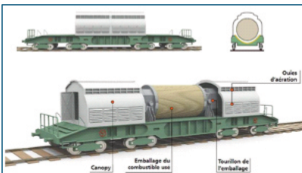
Figure 3. Château de transport de combustible usé (source : EDF)
