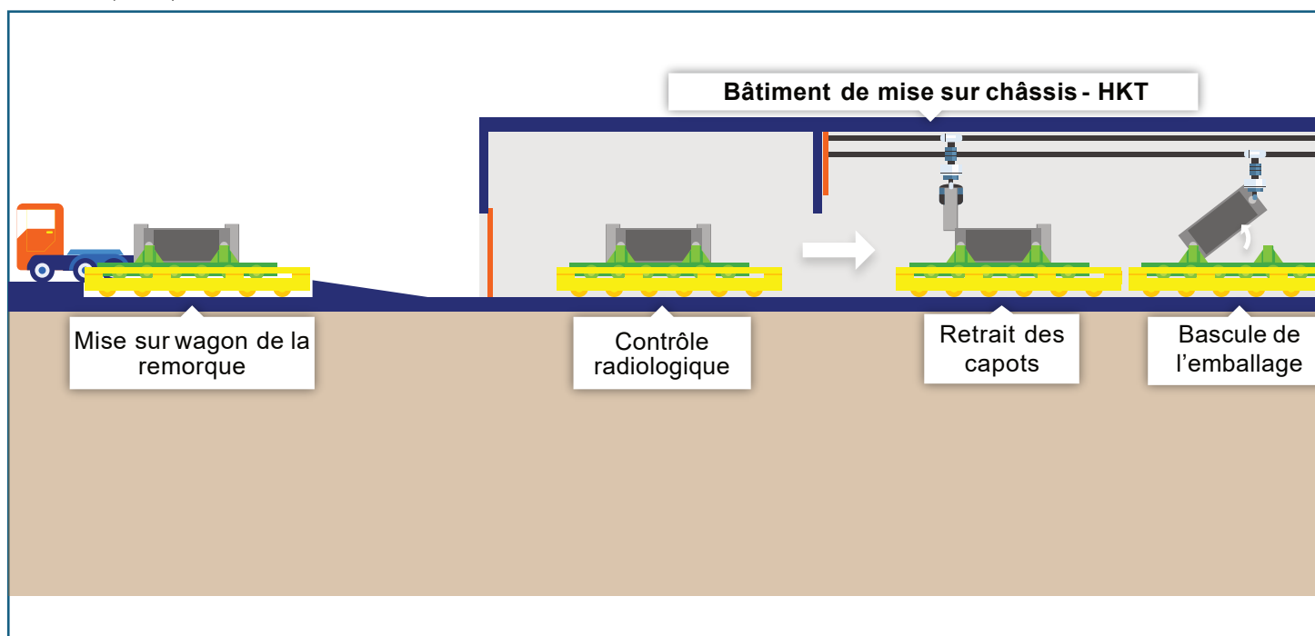
Figure 7. Schéma présentant le parcours d'un assemblage combustible et quelques-unes
