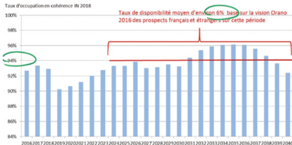
Figure 9. Évolution du taux d'occupation des piscines de la Hague - Présentation d'Orano "Enjeux et Perspectives" au HCTISN
