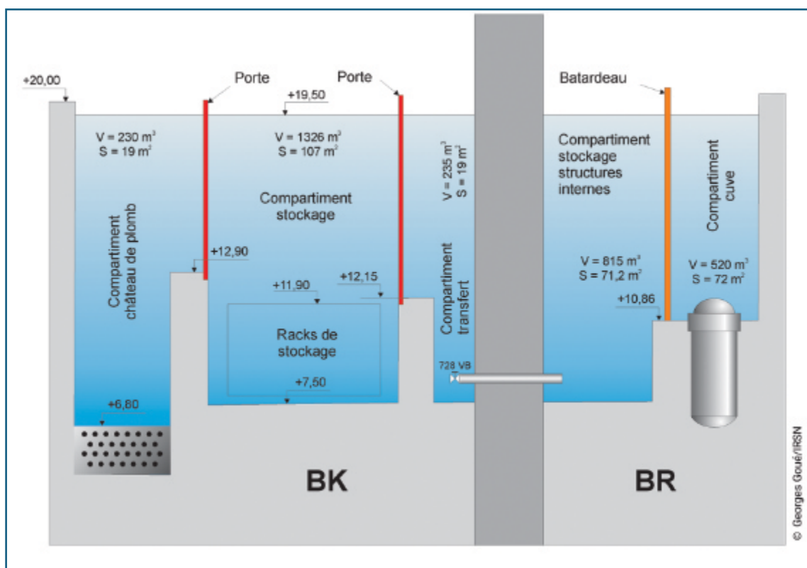
Figure 4. Schéma des piscines d'un bâtiment combustible (BK) et d'un bâtiment réacteur (BR) (source : IRSN)
