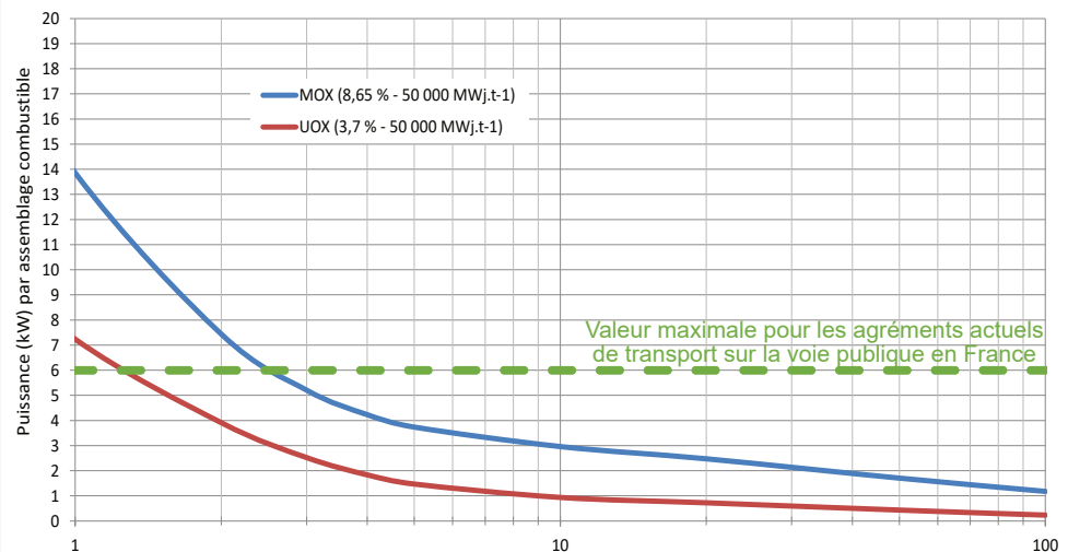
Figure 2. Courbes de décroissance de la puissance thermique d'un assemblage de combustible UOX et d'un assemblage de combustible MOX, irradiés dans un réacteur français (source : rapport IRSN n° 2018-00003)
