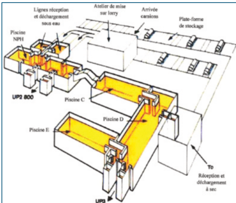
Figure 6. Schéma des piscines de l'usine d'Orano La Hague (source : rapport IRSN n° 2018-00003)
