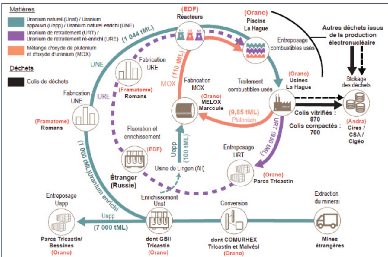
Figure 1. « Cycle du combustible » en France (source : Rapport de la Cour des Comptes « L'aval du cycle du combustible nucléaire ») - Note : les flux indiqués correspondent aux flux de l'année 2017. Les flèches en pointillés correspondent à des étapes non-opérationnelles en 2017.
